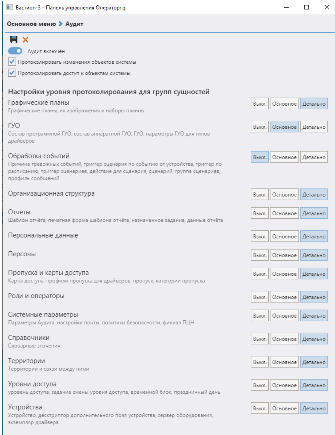
Рис. 1. Настройка модуля «Бастиян-3 — Аудит системы»
